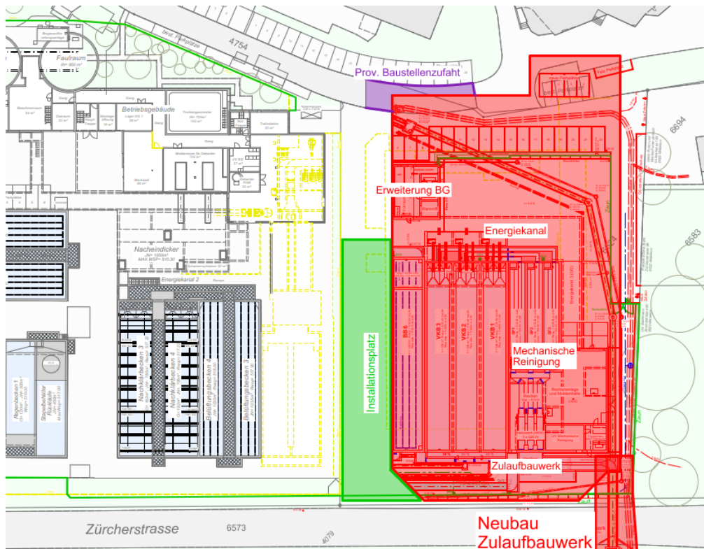
Ausbau ARA Flos; Etappe Mechanische Reinigung
