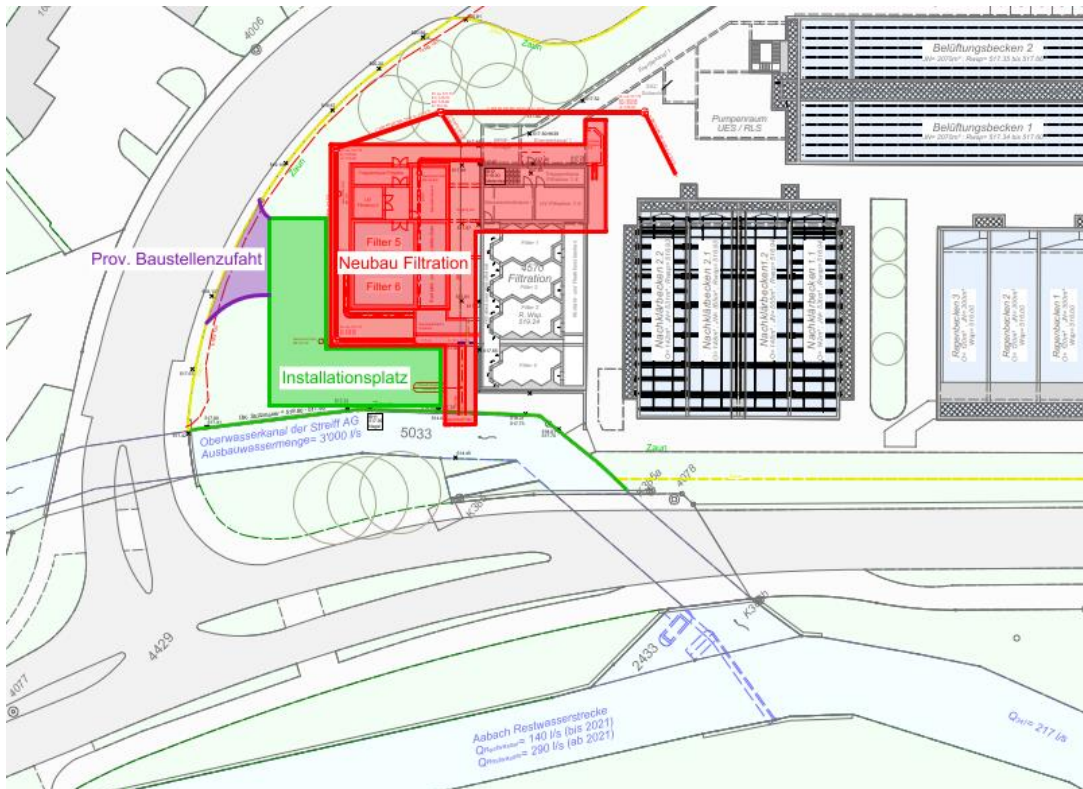
Ausbau ARA Flos; Etappe Erweiterung Filtration
